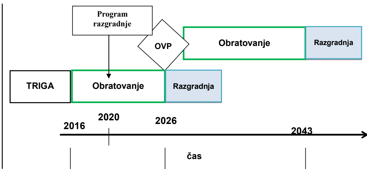
Slika 8: Shematski prikaz glavnih mejnikov strategije 7
