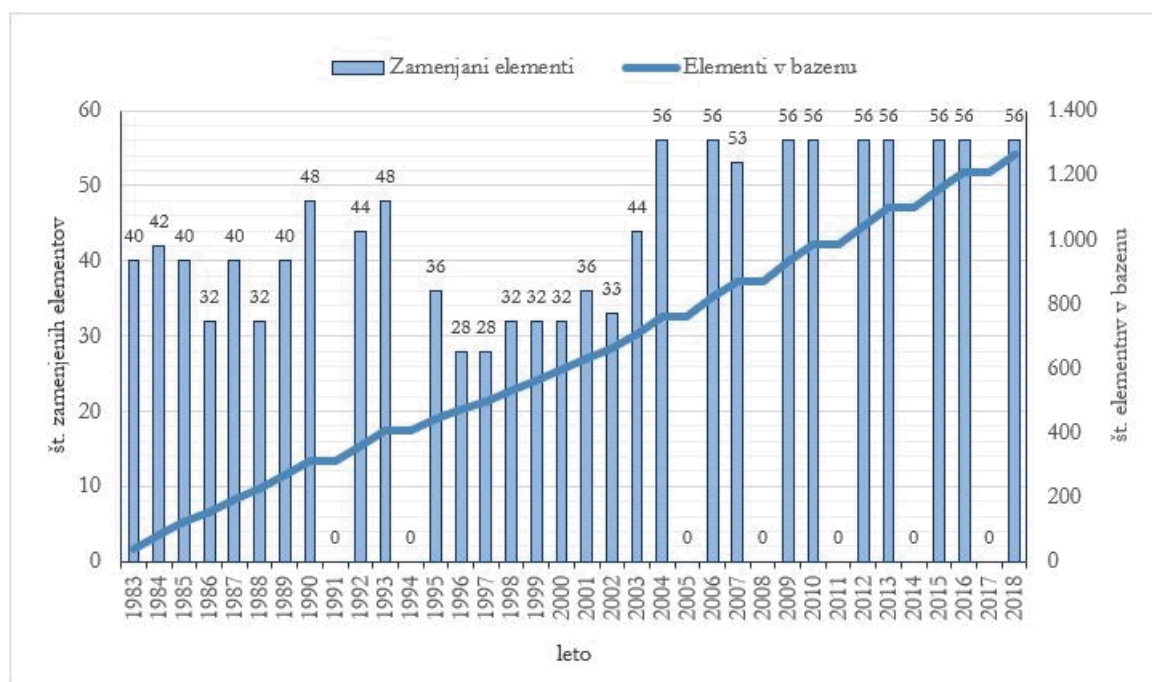
Slika 17: Število letno zamenjanih izrabljenih gorivnih elementov in število vseh takih elementov v bazenu NEK
