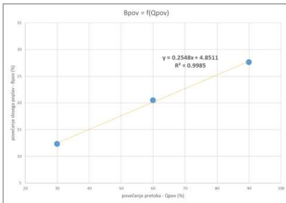
Slika 191. Prikaz odvisnosti povečanja dosega poplav od povečanja pretoka
