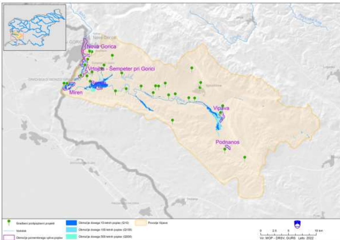
Slika 165. Prikaz porečja Vipave z lokacijami gradbenih protipoplavnih ukrepov (informativni prikaz).
