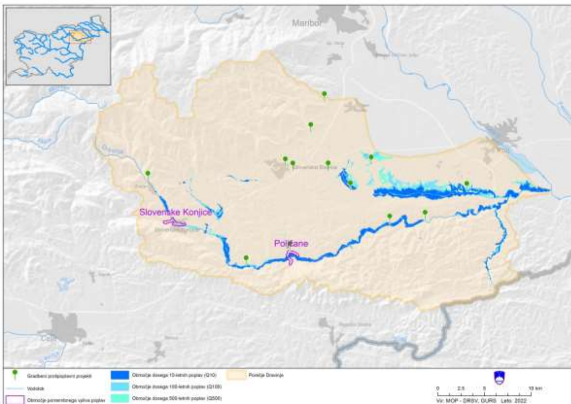
Slika 126. Prikaz porečja Dravinje z lokacijami gradbenih protipoplavnih ukrepov (informativni prikaz).
