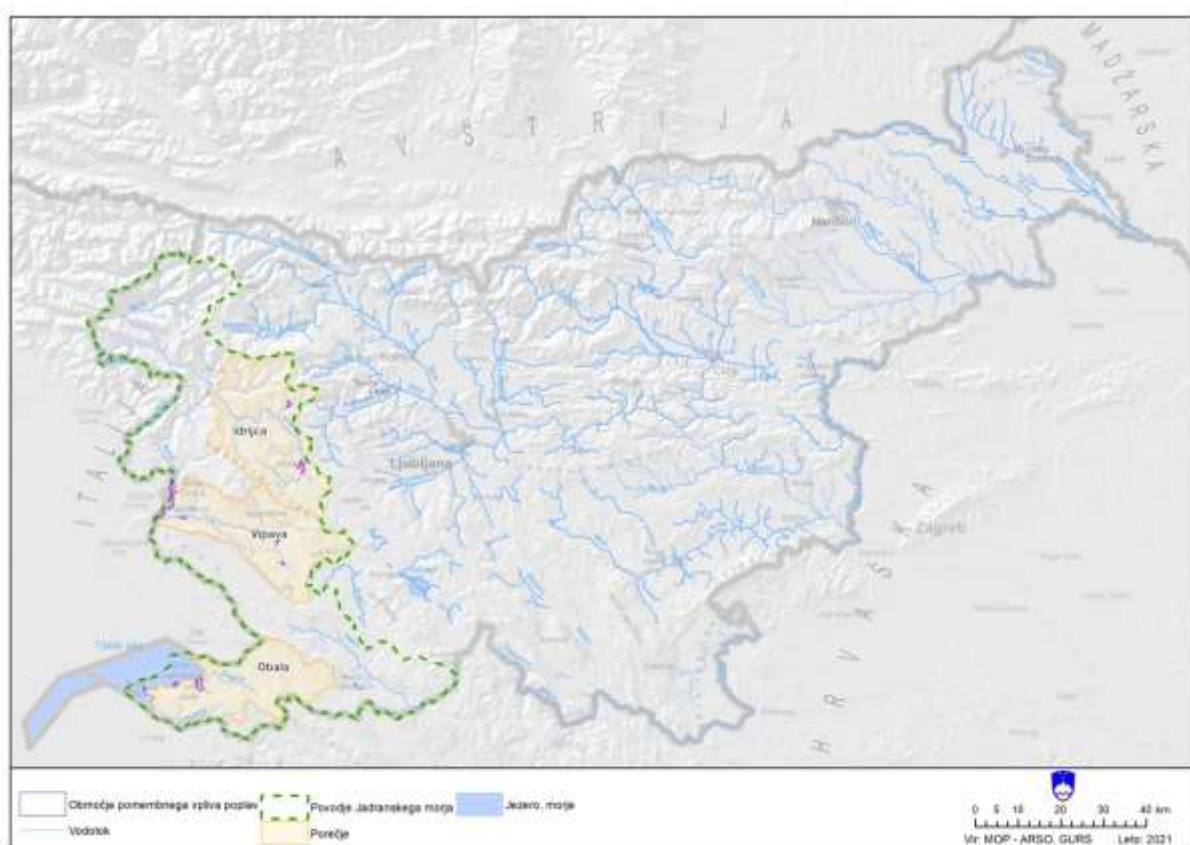
Slika 147. Območja pomembnega vpliva poplav na območju povodja Jadranskega morja.
