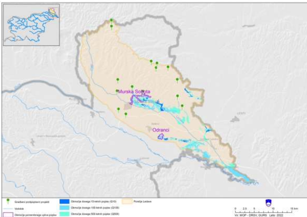
Slika 145. Prikaz porečja Ledave z lokacijami gradbenih protipoplavnih ukrepov (informativni prikaz).
