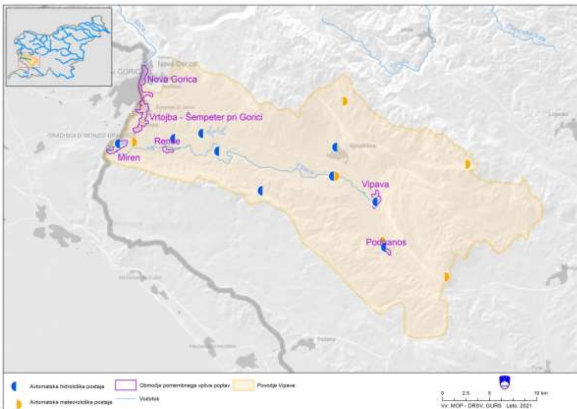
Slika 164. Prikaz lokacij hidrološkega in meteorološkega monitoringa na porečju Vipave.
