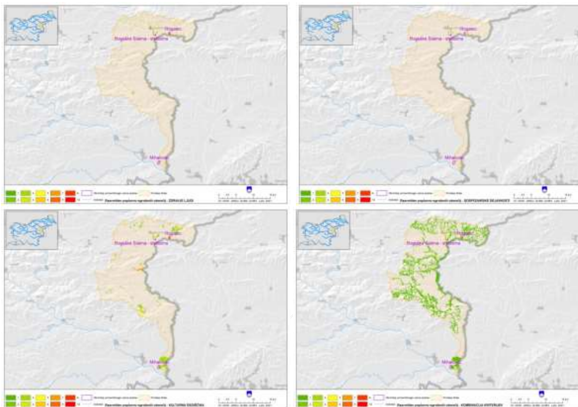
Slika 84. Ugotovitve iz predhodne ocene poplavne ogroženosti – razvrstitev poplavno ogroženih območij na porečju Sotle po kriterijih zdravlja ljudi, gospodarskih dejavnosti, kulturne dediščine in skupne kombinacije vseh kategorij (zeleno – najmanj ogroženo; rdeče – najbolj ogroženo).
