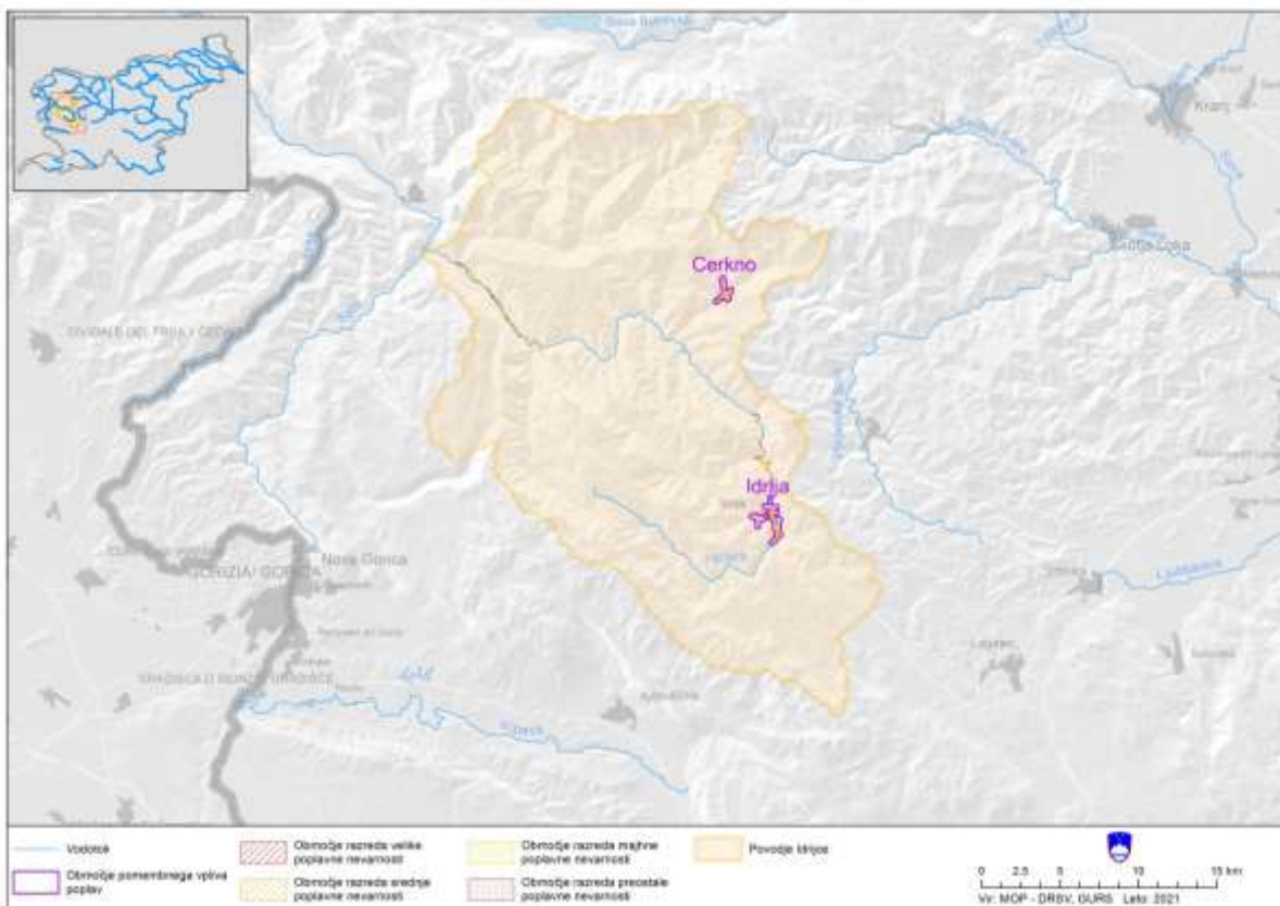
Slika 152. Prikaz razredov poplavne nevarnosti (velika, srednja, majhna in preostala) na porečju Idrijce.
