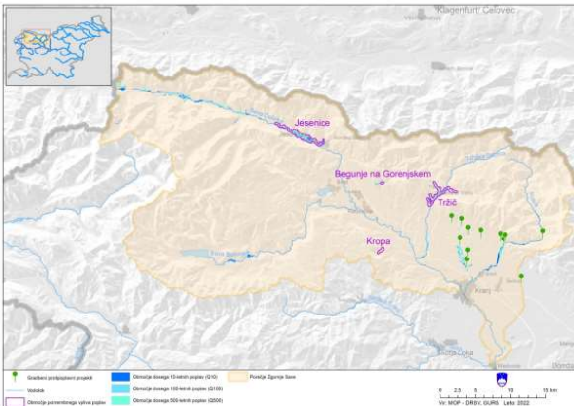
Slika 18. Prikaz porečja Zgornje Save z lokacijami gradbenih protipoplavnih ukrepov (informativni prikaz).
