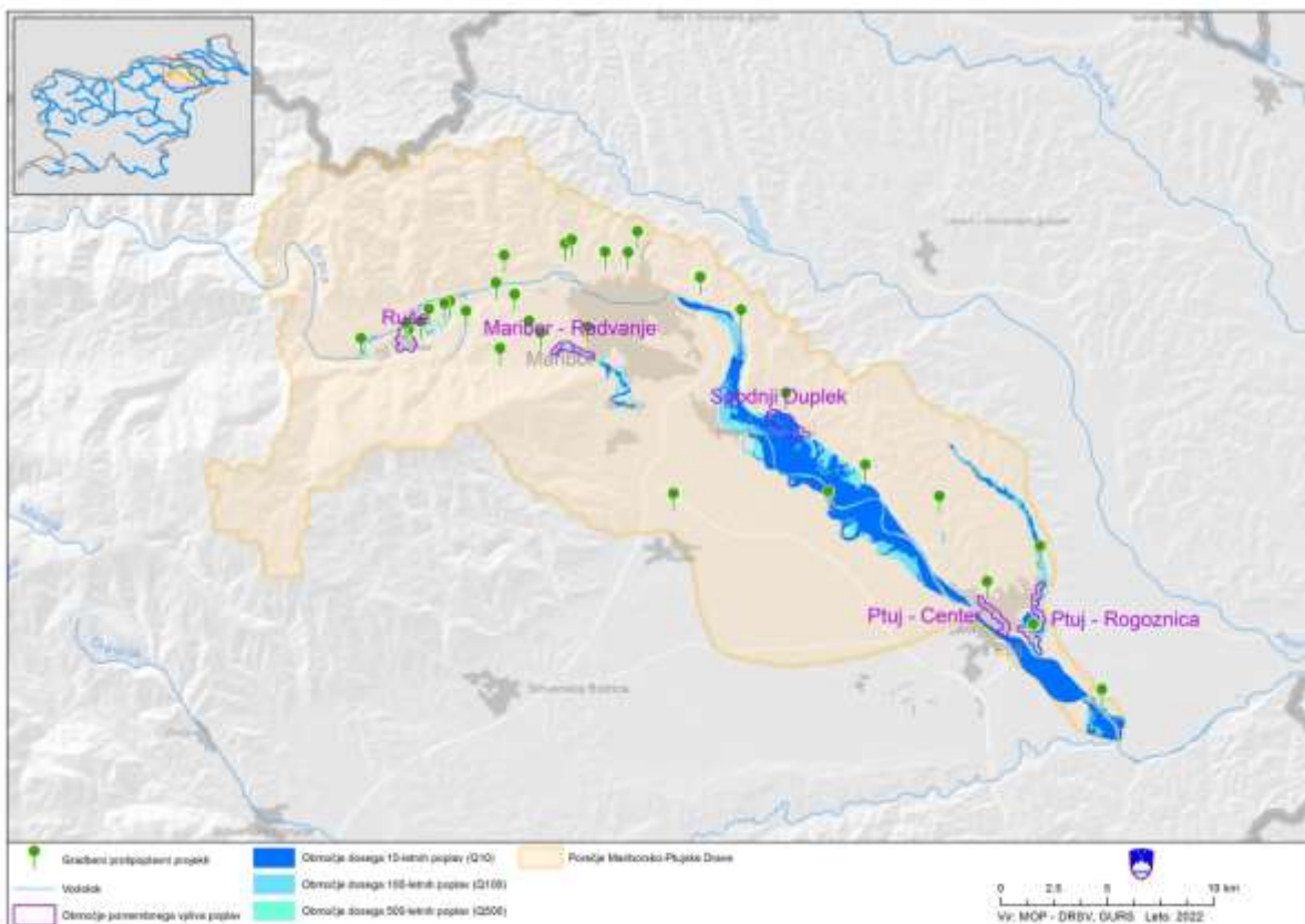
Slika 117. Prikaz porečja Mariborsko-Ptujske Drave z lokacijami gradbenih protipoplavnih ukrepov (informativni prikaz).
