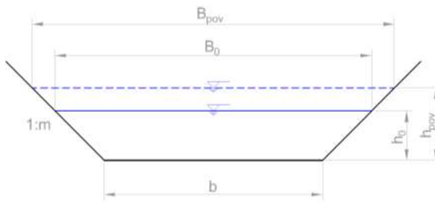
Slika 190. Karakteristični prikaz testnega pretočnega korita
