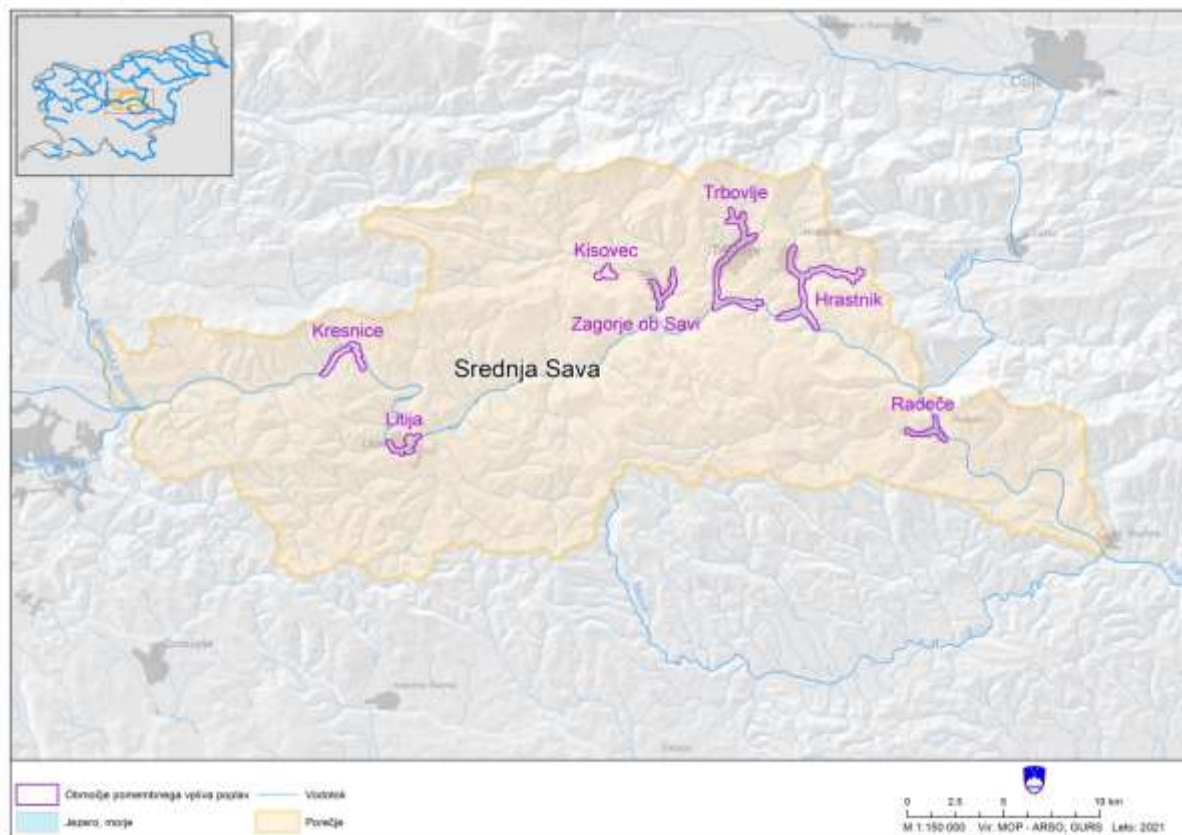
Slika 56. Prikaz porečja Srednje Save z lokacijami območij pomembnega vpliva poplav.
