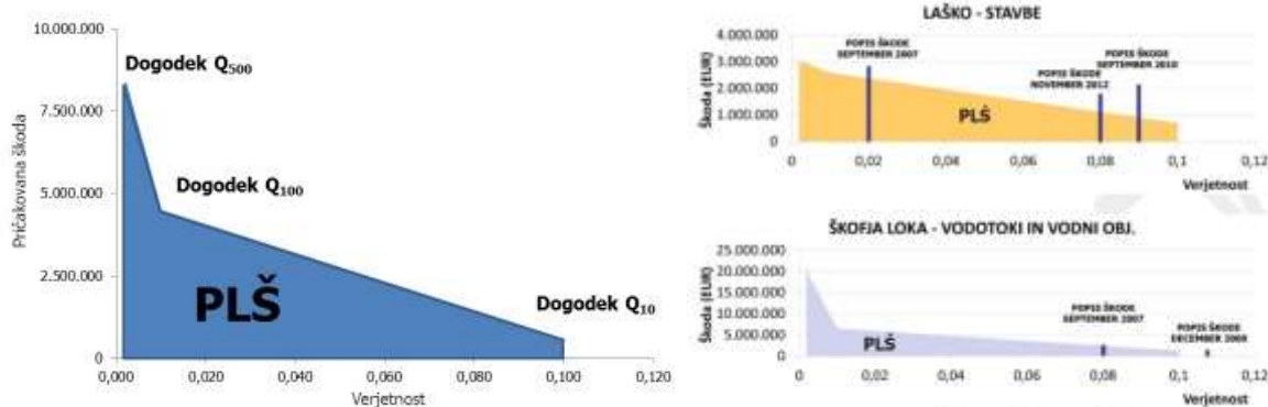
Slika 178. Izračun pričakovane letne škode pred izvedbo ukrepov (levo) in primerjava izračunane pričakovane škode s popisano škodo pri preteklih poplavnih dogodkih v Laškem in Škofji Loki (desno).
