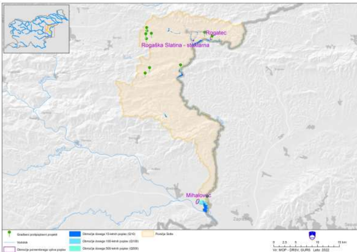
Slika 90. Prikaz porečja Sotle z lokacijami gradbenih protipoplavnih ukrepov (informativni prikaz).
