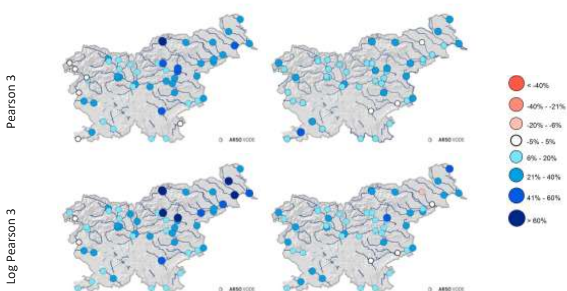
Slika 188. Sprememba pretokov stoletnih (Q100) povratnih dob v obdobjih 2011–2040 (levo) in 2041–2070 (desno) v primerjavi z obdobjem 1981–2010, po scenariju izpustov toplogrednih plinov RCP4.5 za porazdelitvi Pearson 3 (zgoraj) in Log Pearson 3 (spodaj)
