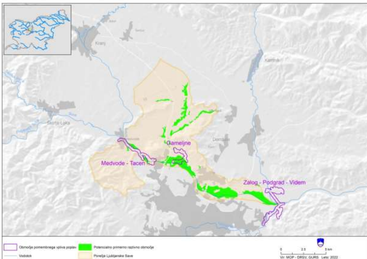
Slika 33. Prikaz lokacij potencialnih območij za razlivanje visokih voda na porečju Ljubljanske Save.
