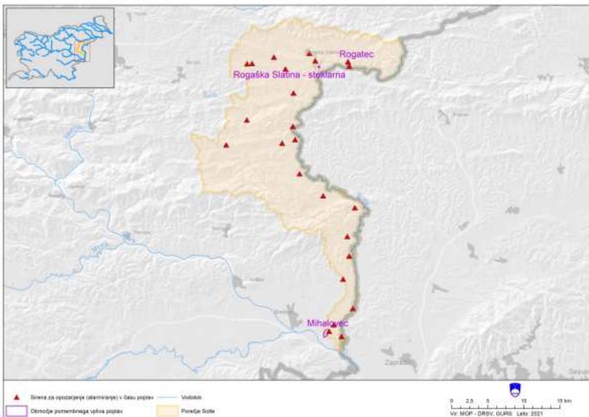
Slika 91. Prikaz porečja Sotle z lokacijami siren za alarmiranje.
