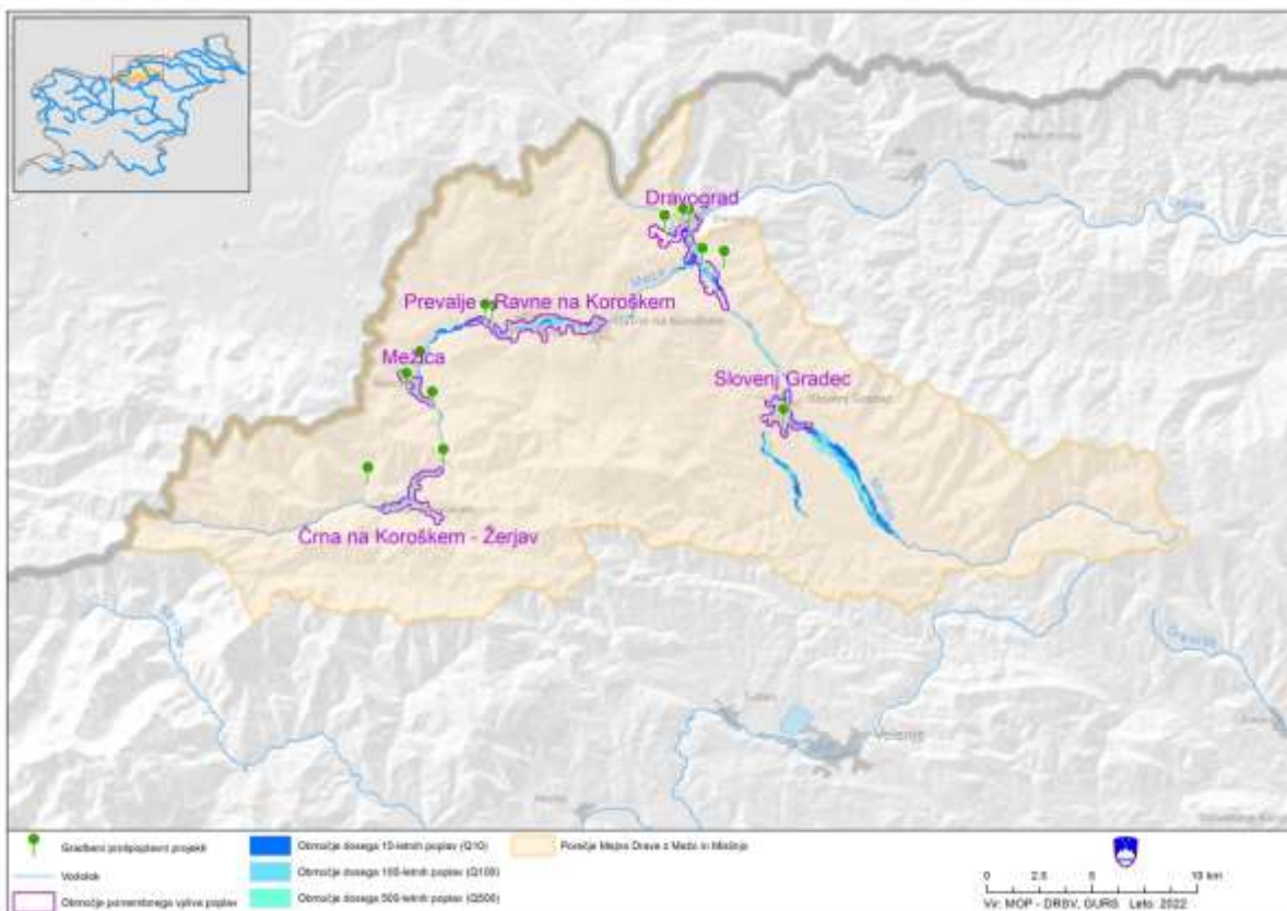
Slika 108. Prikaz porečja Mejne Drave z Mežo in Mislinjo z lokacijami gradbenih protipoplavnih ukrepov (informativni prikaz).
