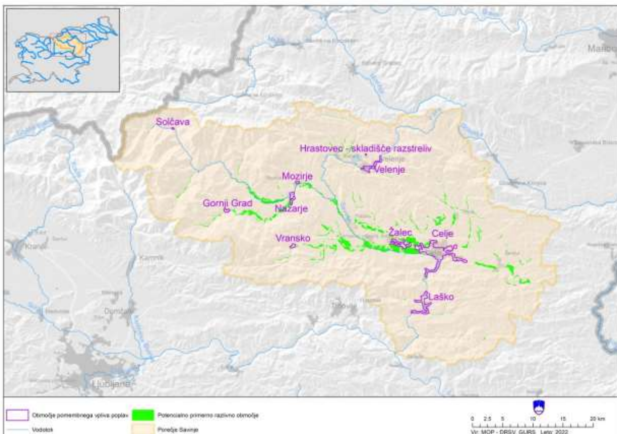
Slika 69. Prikaz lokacij potencialnih območij za razlivanje visokih voda na porečju Savinje.
