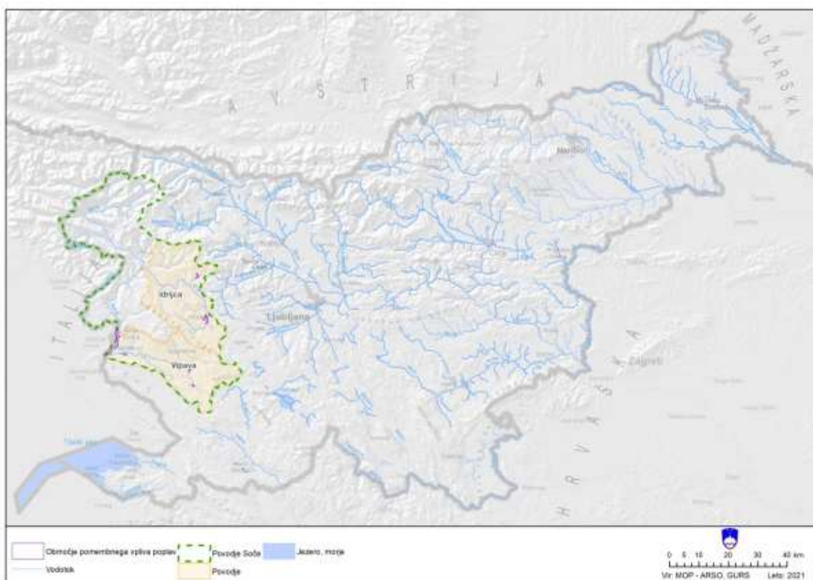
Slika 148. Območja pomembnega vpliva poplav na območju povodja Soče.
