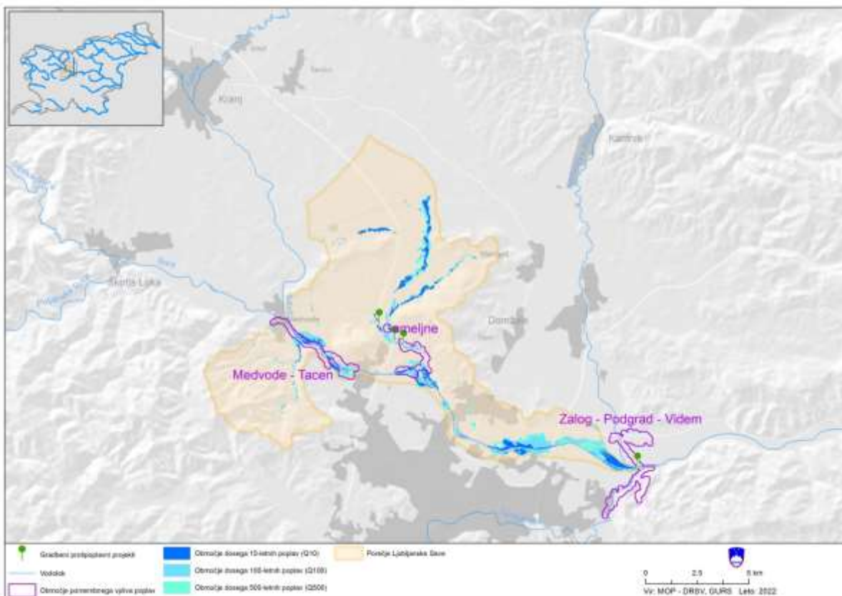
Slika 36. Prikaz porečja Ljubljanske Save z lokacijami gradbenih protipoplavnih ukrepov (informativni prikaz).
